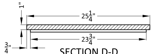
SECTION D-D
